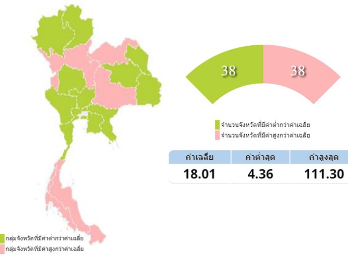
สัดส่วนการปล่อยก๊าซเรือนกระจกต่อผลิตภัณฑ์มวลรวมฯ(รายจังหวัด)
