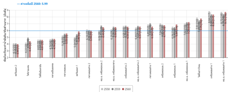
สัดส่วนการใช้พลังงานขั้นสุดท้ายต่อผลิตภัณฑ์มวลรวมฯ (รายภาค)
