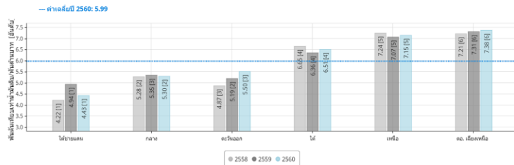
สัดส่วนการใช้พลังงานขั้นสุดท้ายต่อผลิตภัณฑ์มวลรวมฯ (รายภาค)
