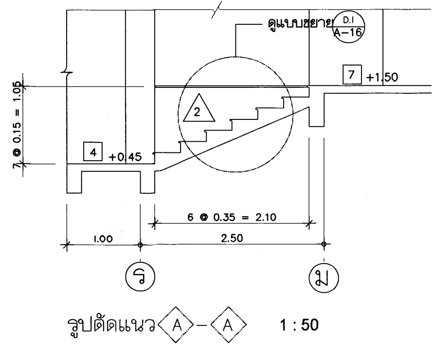
แปลนบันได ST4 18 50
