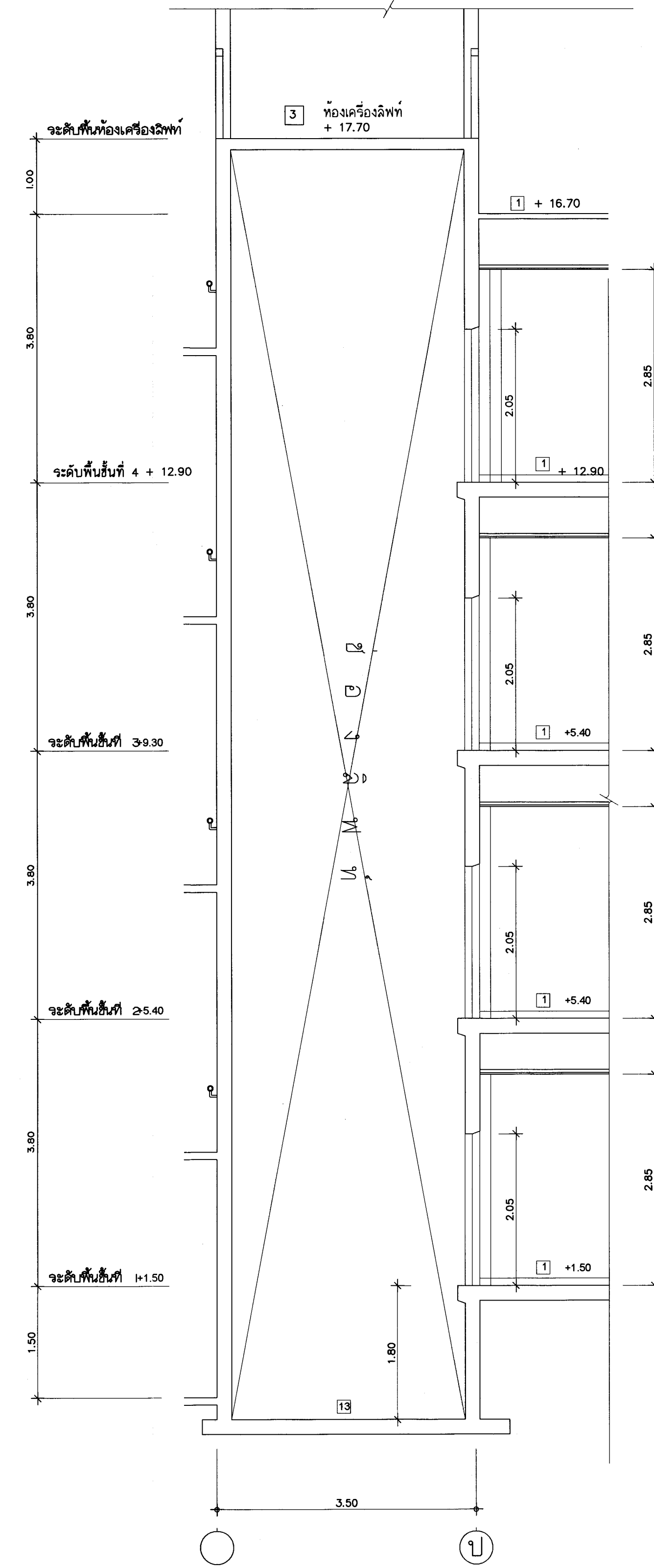
รูปตัดแนว B - B 1:50
