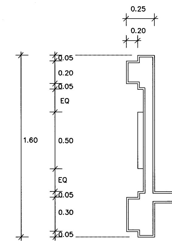
รูปตัดขยาย 4 : 1 : 20
