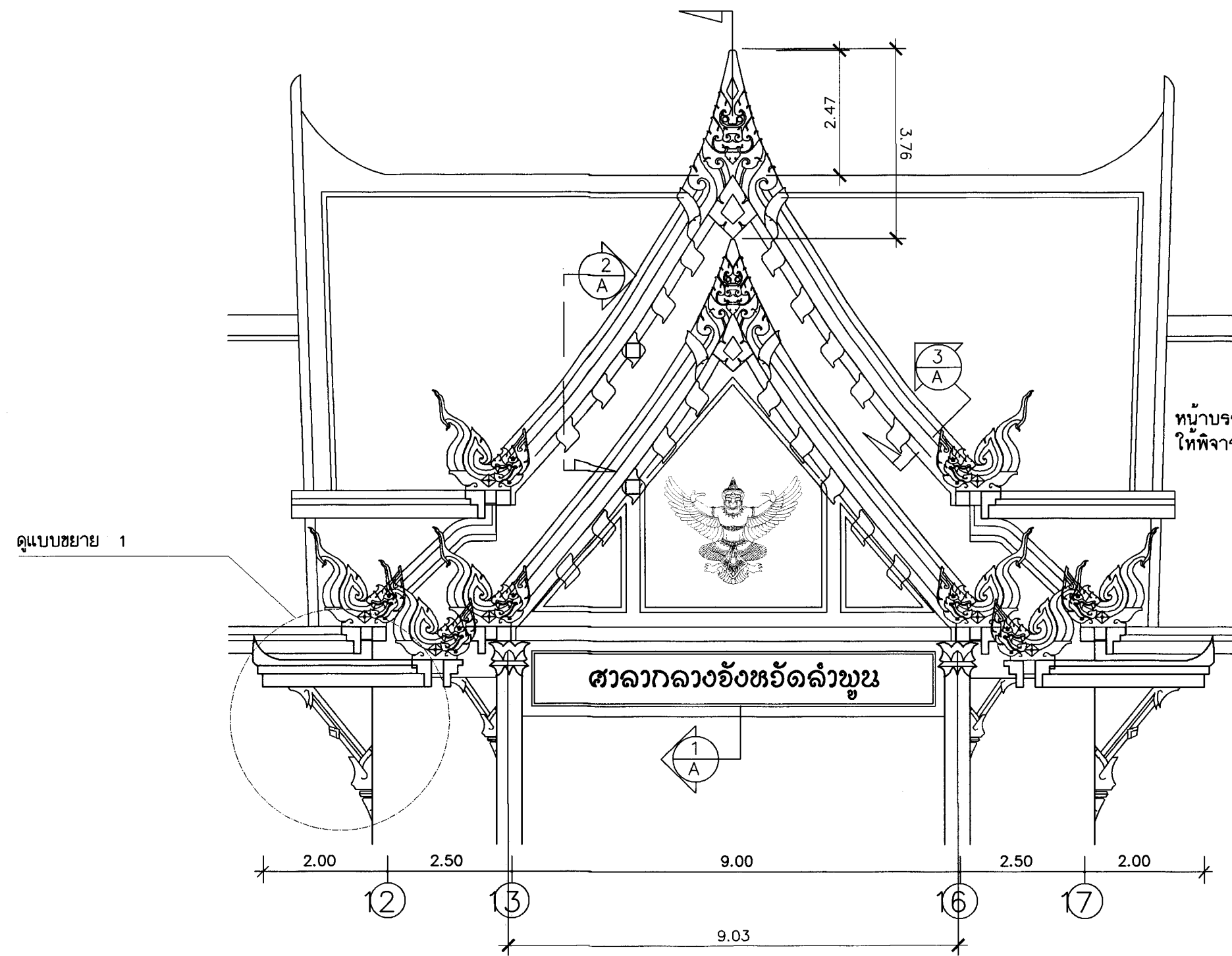
ขยายหน้าจั่ว 1 : 100
