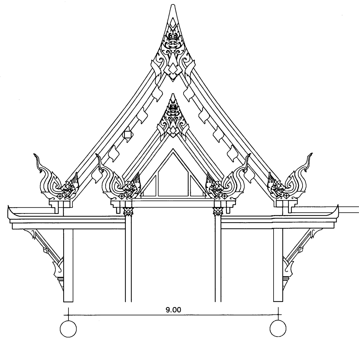
ขยายหน้าจั่ว 1 : 100
