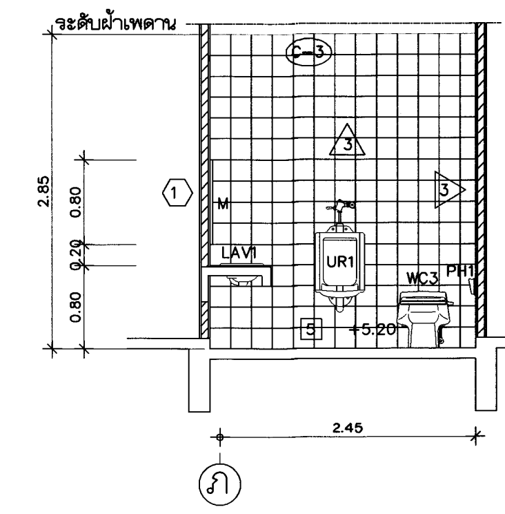
รูปตัด D 1:50
