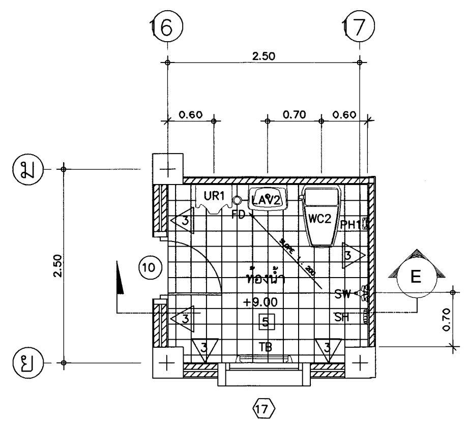
แปลนห้องน้ำ 11 ๘ 1 50
