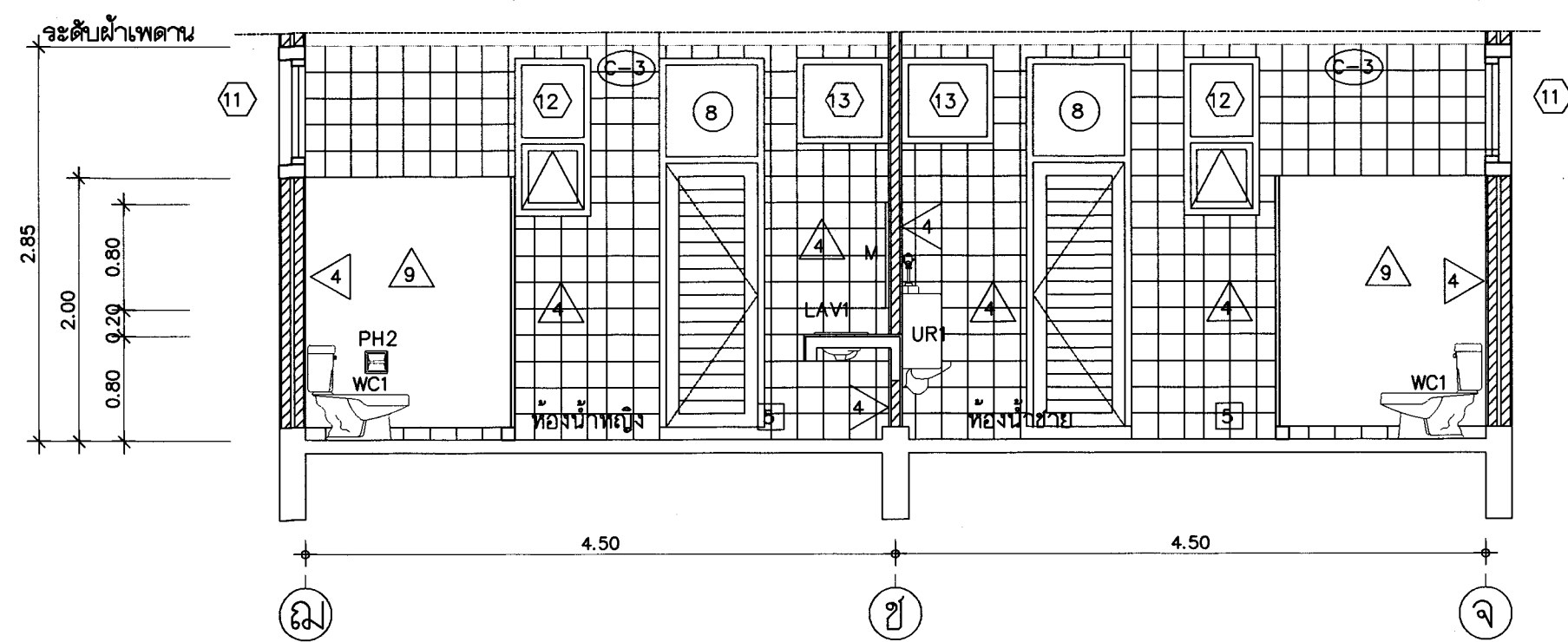
รูปตัด A 1:50
