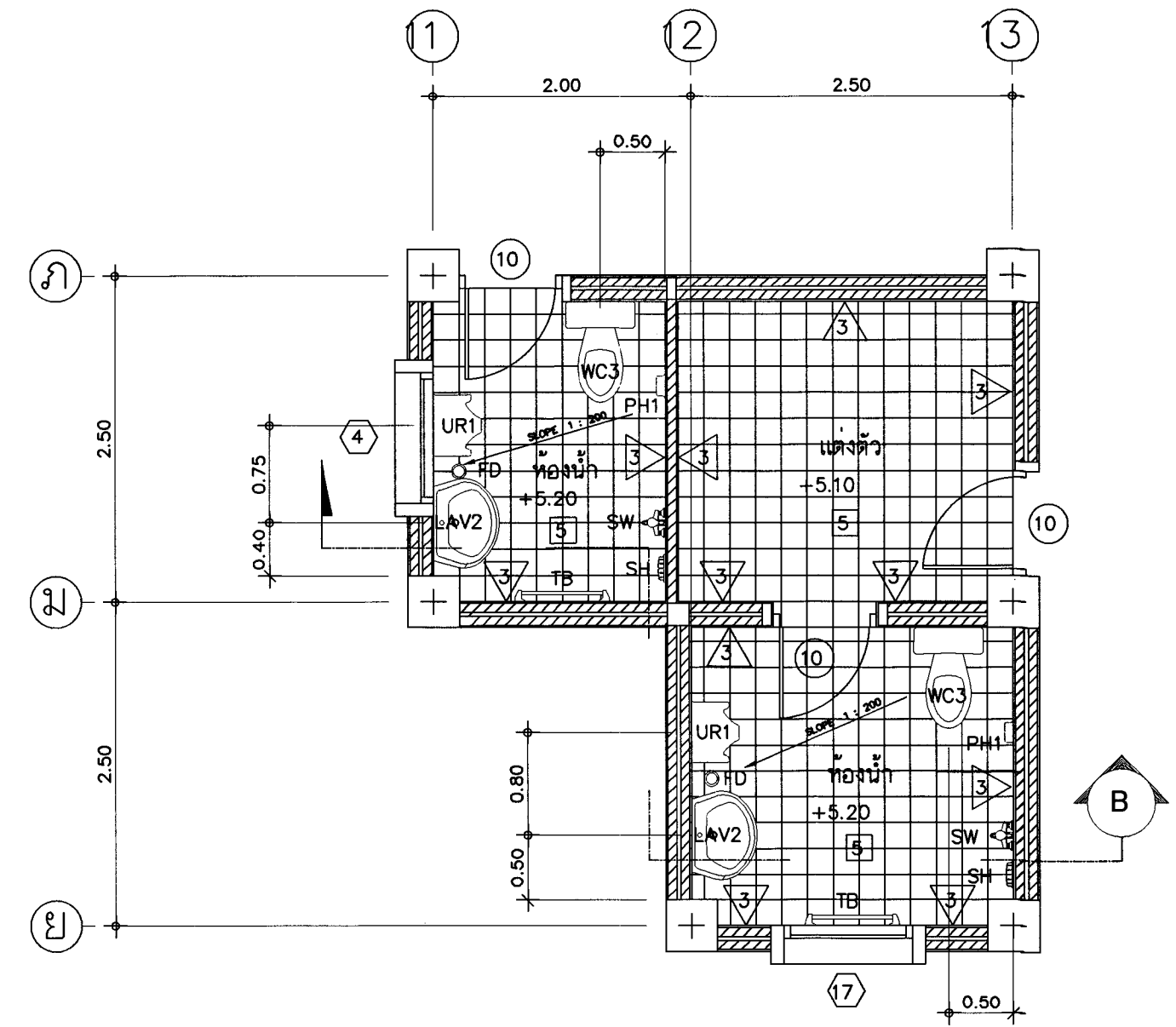
แปลนห้องน้ำ 8 , 8.1 ๘ 1 50
