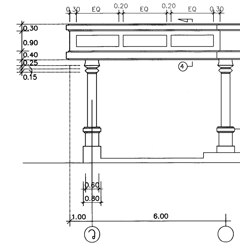
รูปด้านข้าง 1 : 100
