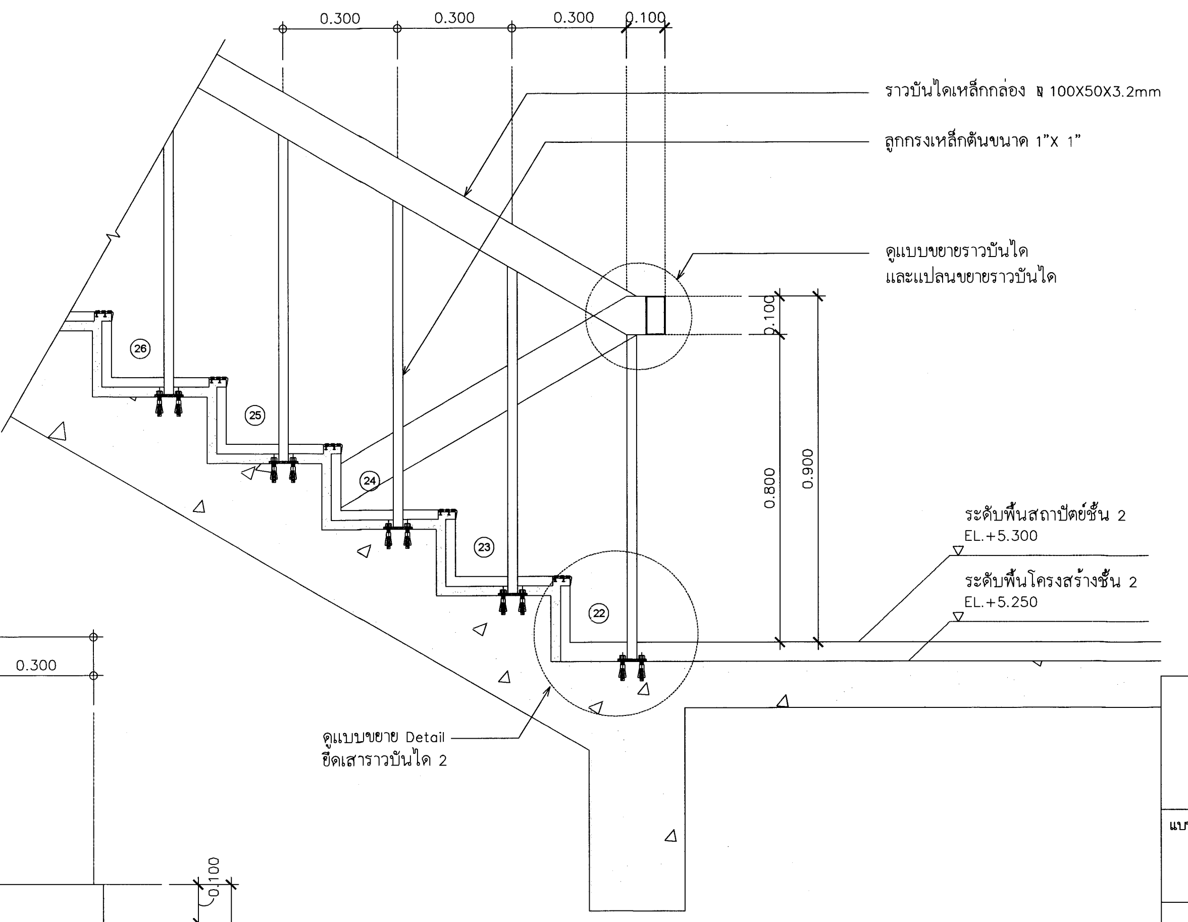
แบบขยายราวบันได มาตราส่วน A1 1:10 A3 1:20
