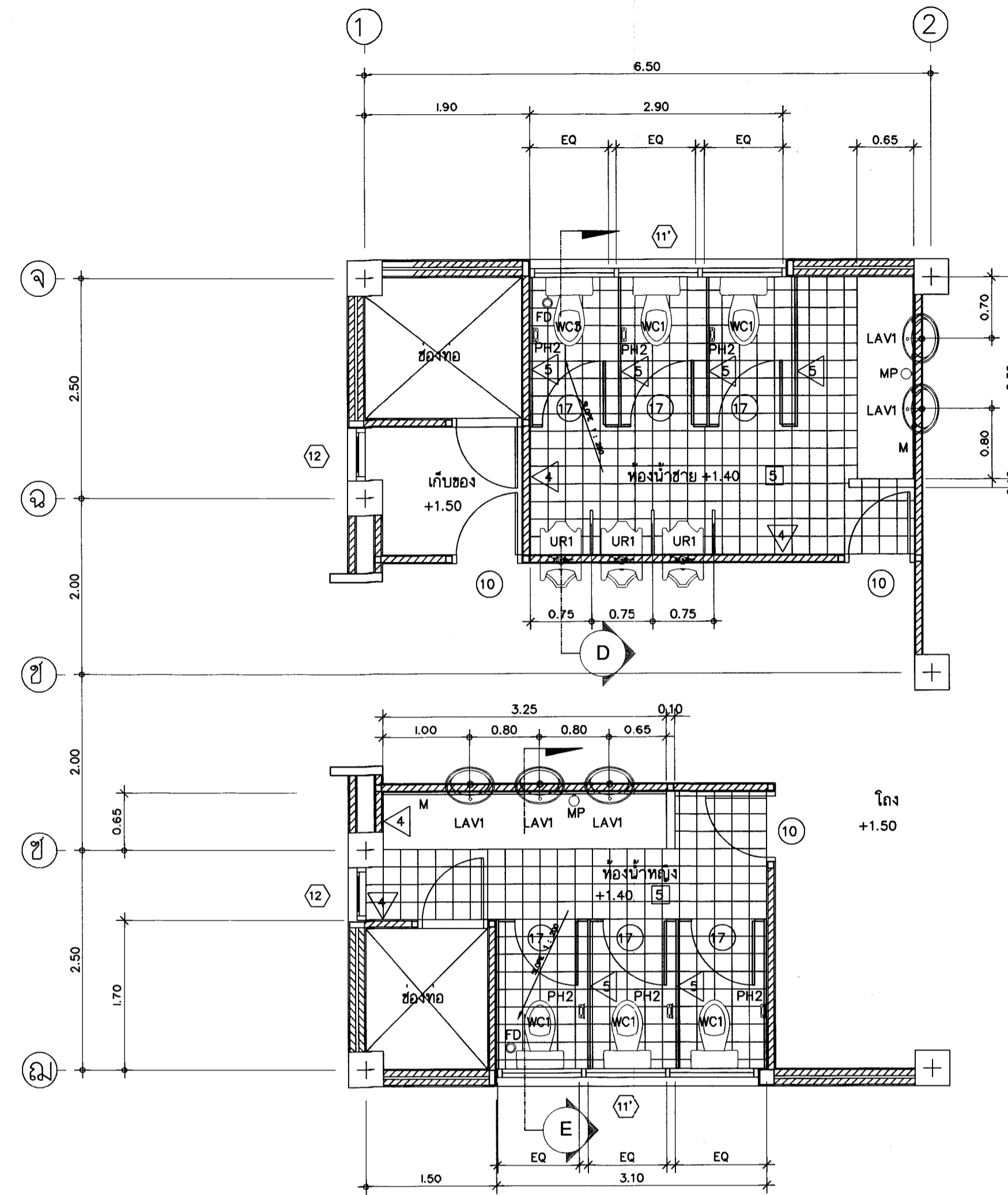
แปลนห้องน้ำ 3, 4 : 1 50
