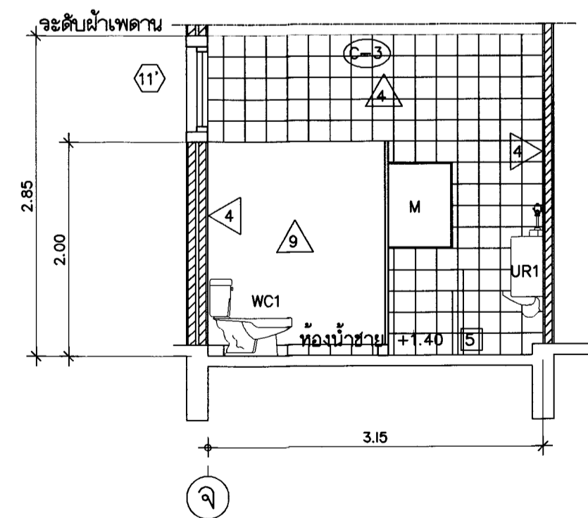
รูปตัด D 1:50
