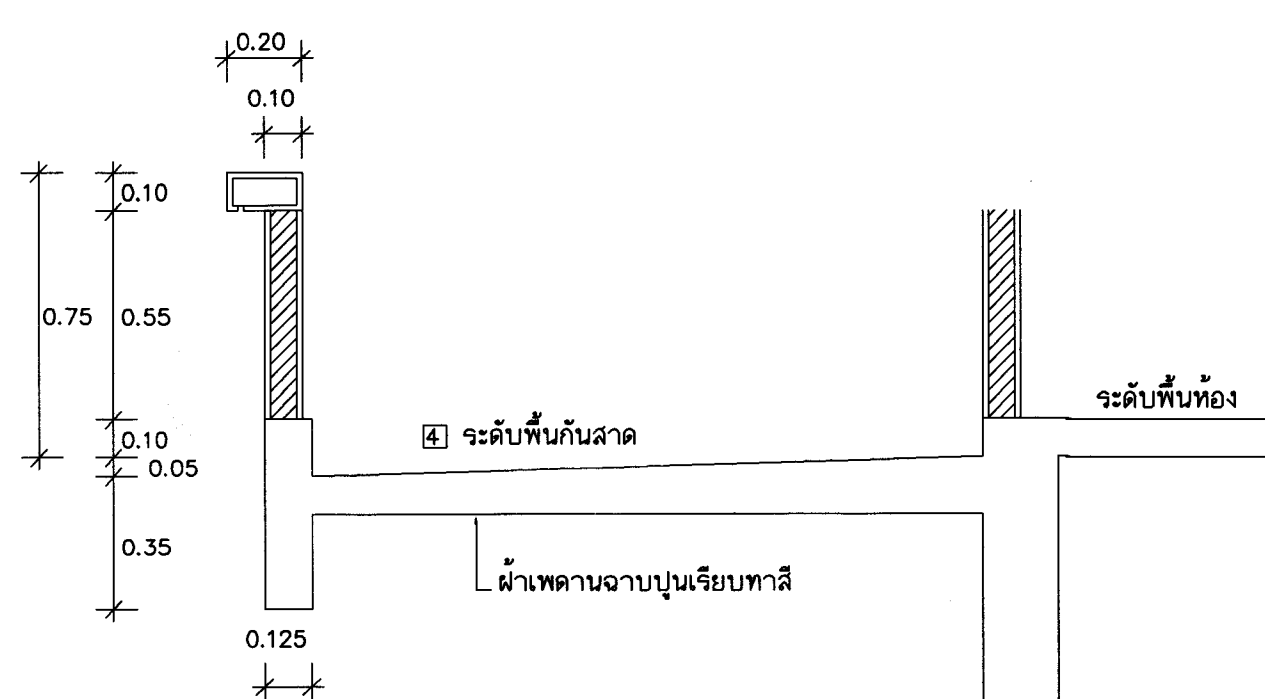
ขยายกันสาด 1 : 20
