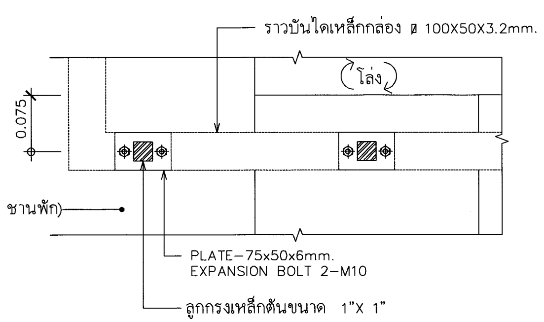
DETAIL ขีดเสาราวบันได 1 SCALE A1 1:5 A3 1:10
