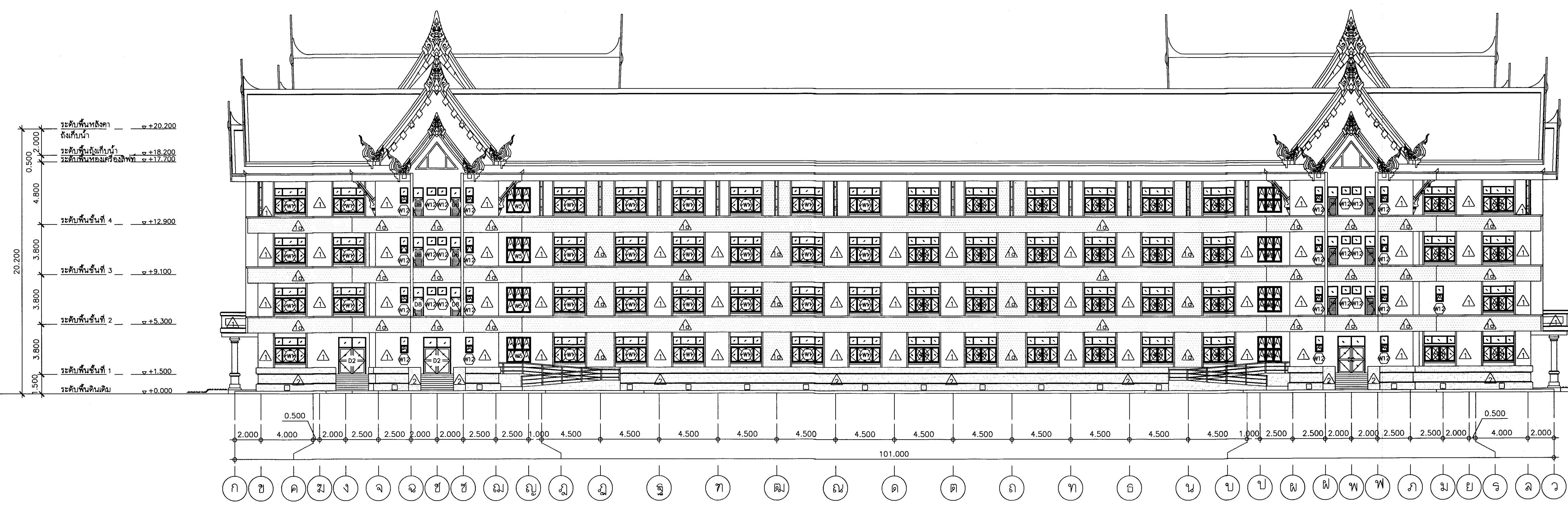
รูปด้าน 2
