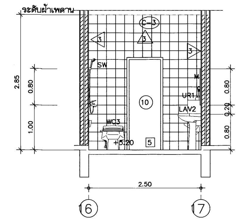
รูปตัด C 1:50
