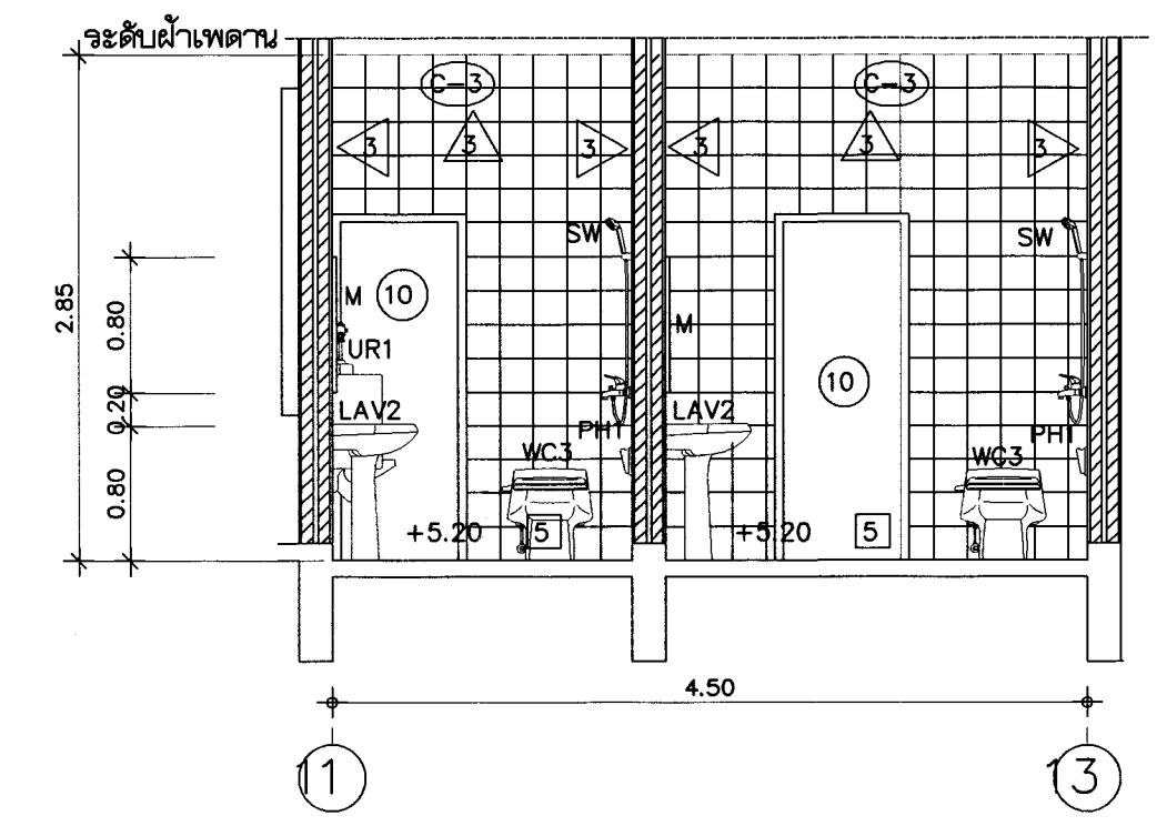
รูปตัด B 1:50
