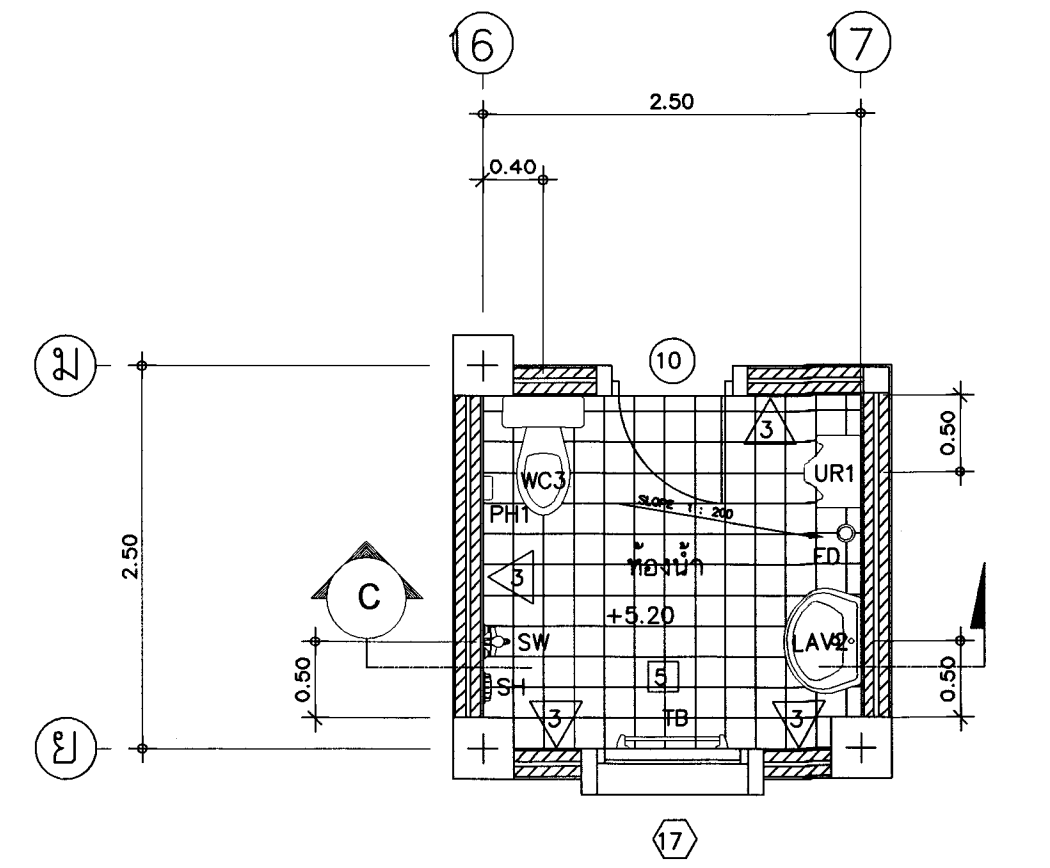
แปลนห้องน้ำ 9 ๘ 1 50
