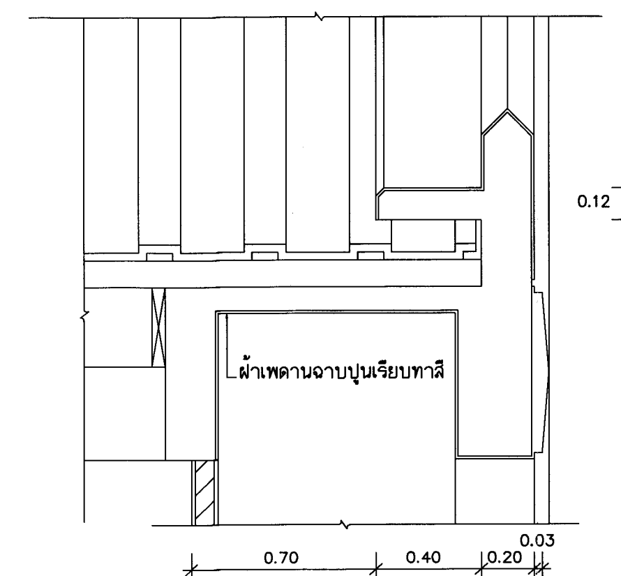
รูปตัด 3 : 1 : 20
