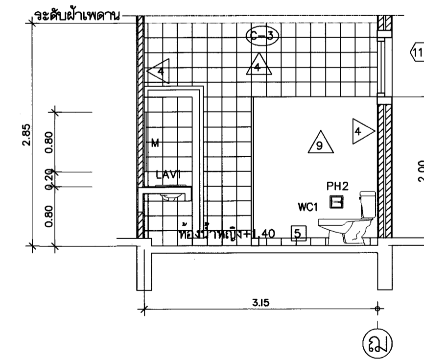
รูปตัด E 1:50
