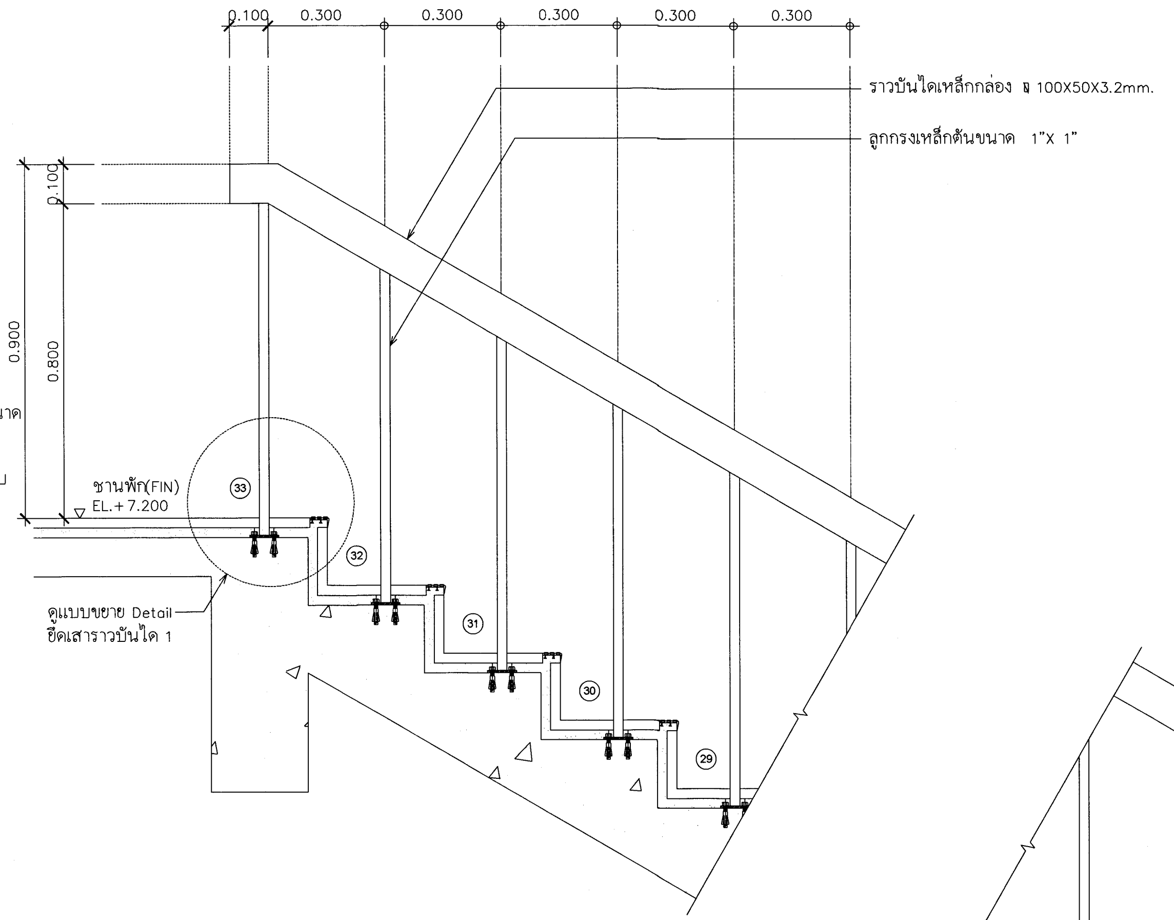
DETAIL A มาตราส่วน A1 1:10 A3 1:20
