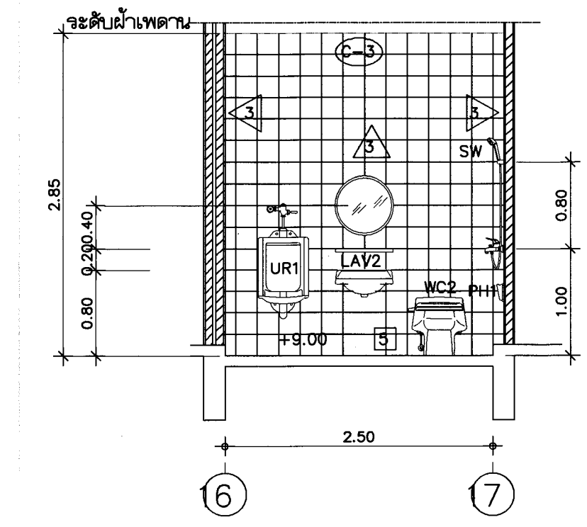
รูปตัด E 1:50
