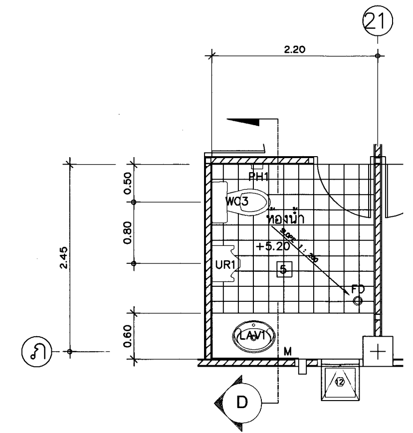
แปลนห้องน้ำ 10 ๘ 1 50
