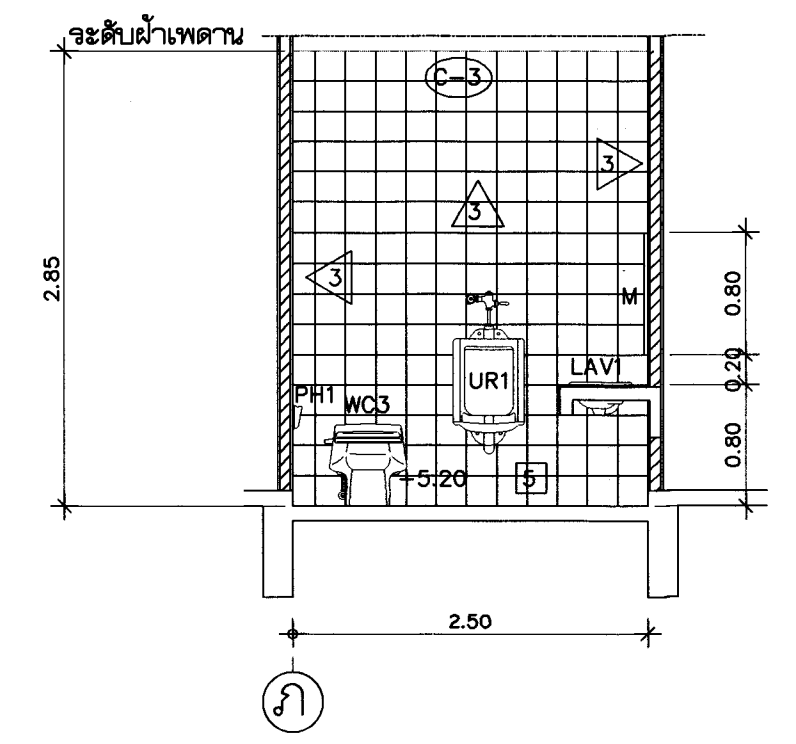
รูปตัด A 1:50
