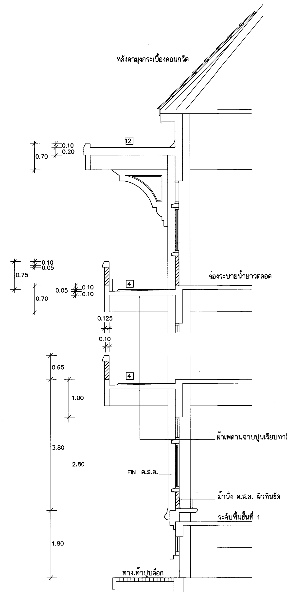
ขยายรูปตัด 1 : 50
