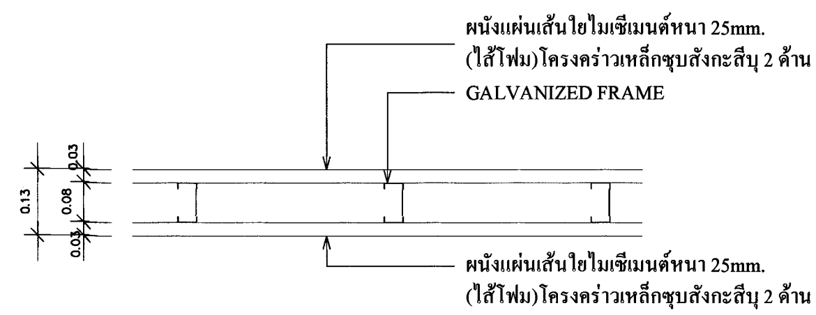
TYPICAL ผนังแผ่นเส้นใยซีเมนต์อัด
