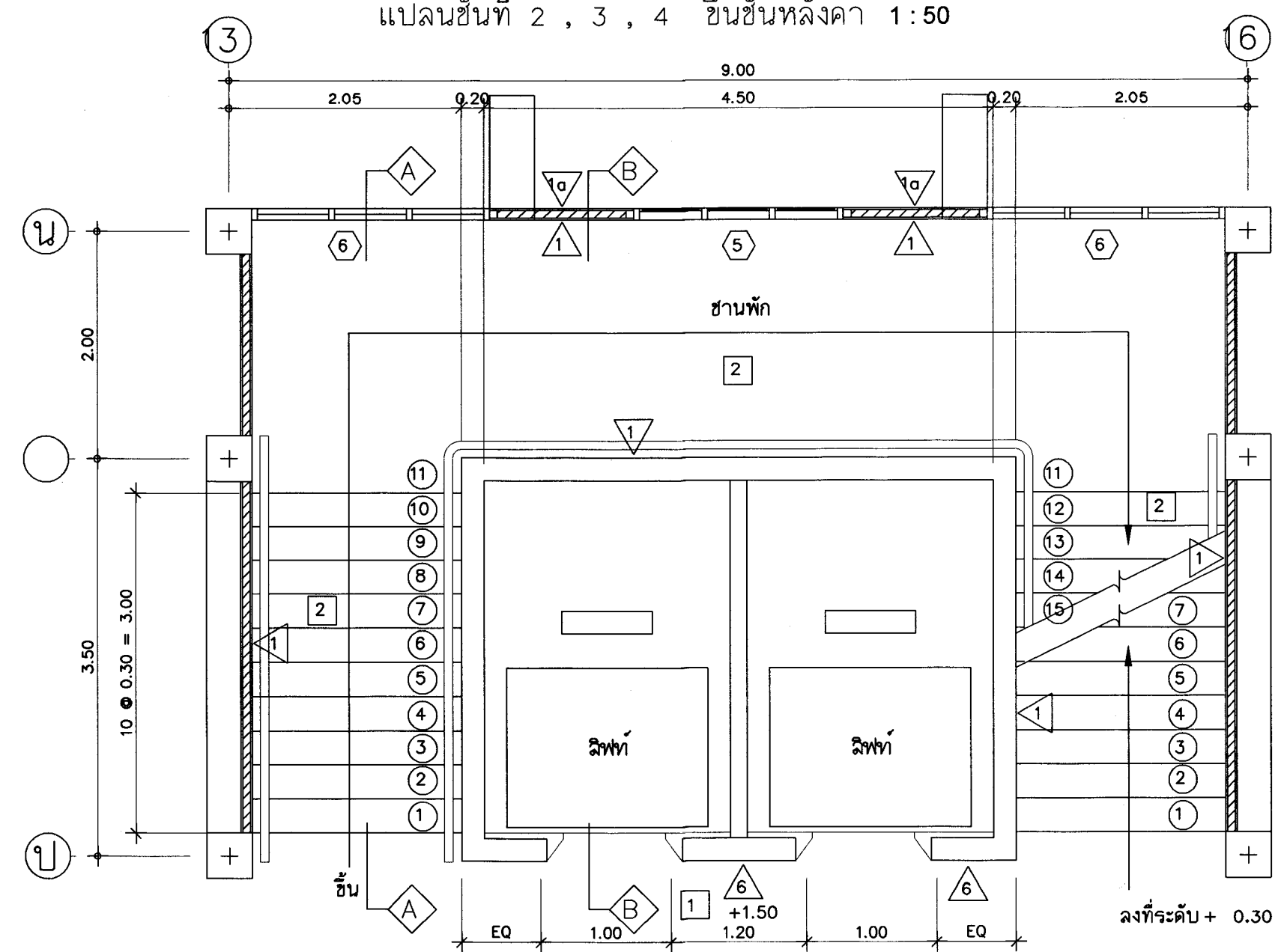
แบบขยายบันได ST.5
