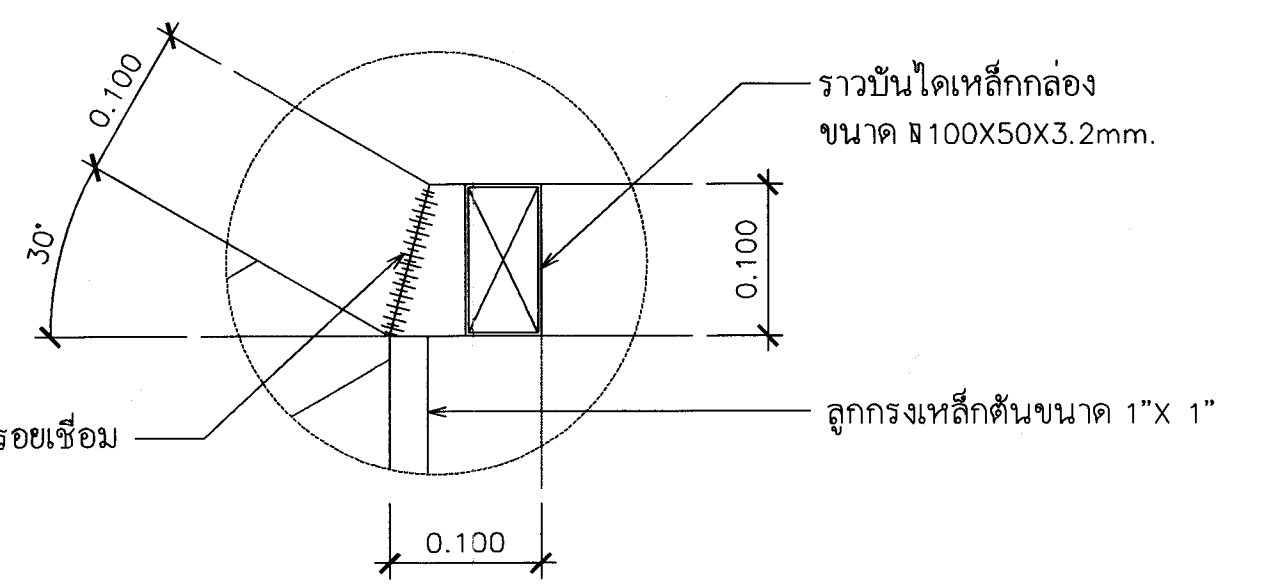
แบบขยายราวบันได มาตราส่วน A3 1:5
