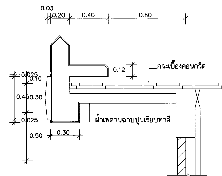
รูปตัด 2 : 1 : 20
