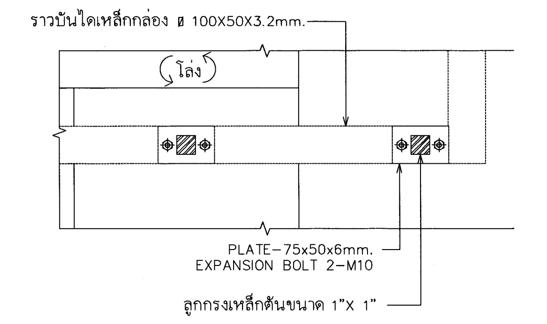
DETAIL ขีดเสาราวบันได 2 SCALE A1 1:5 A3 1:10
