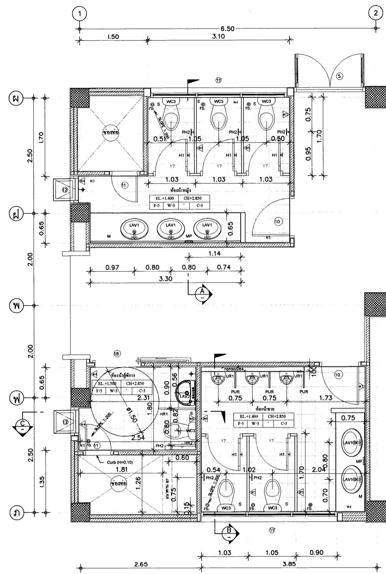
แปลนห้องน้ำ 1, 2 : 1 50
