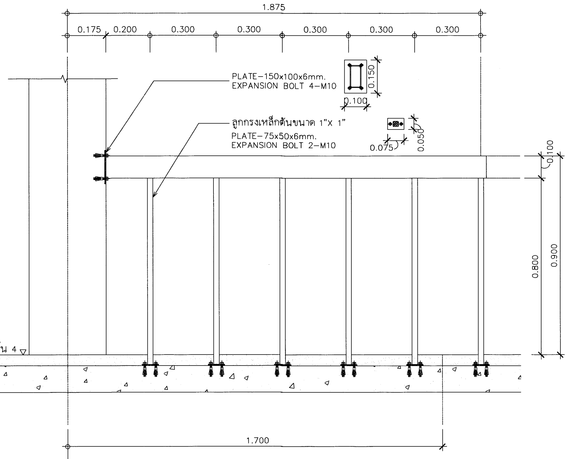
DETAIL C มาตราส่วน A1 1:10 A3 1:20
