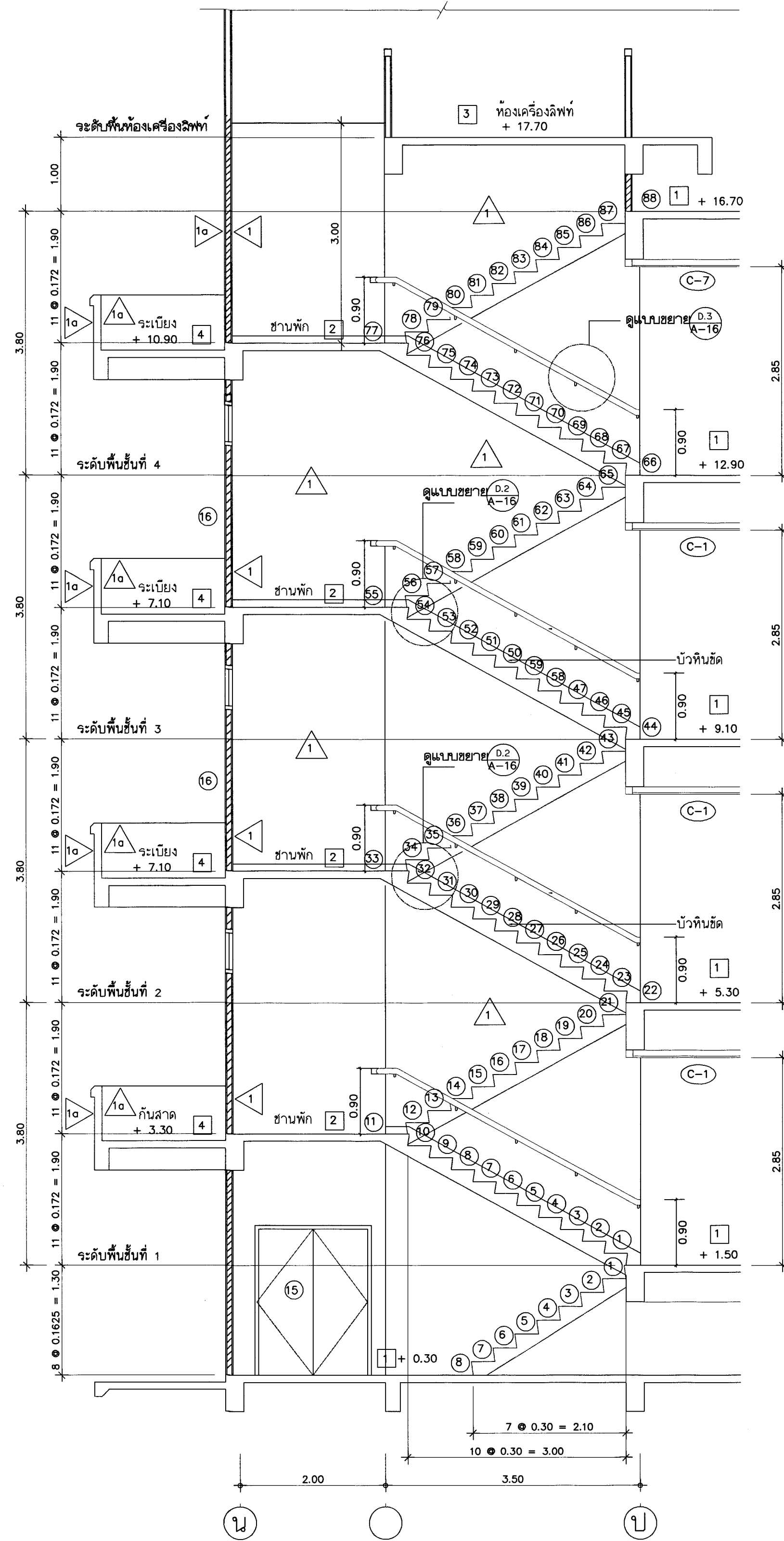
รูปตัดแนว A - A 1:50
