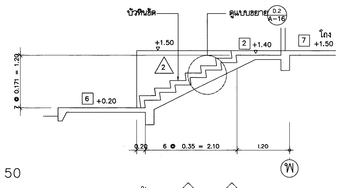
รูปตัดแนว B-B 1:50
